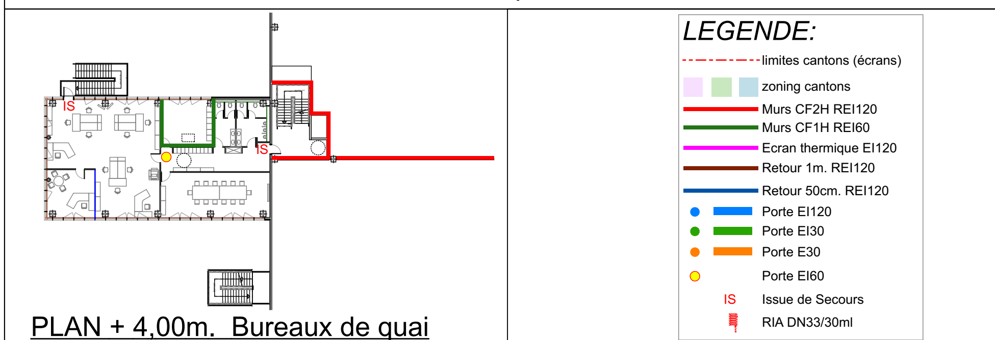
PLAN + 4.00m. Bureaux de quai
